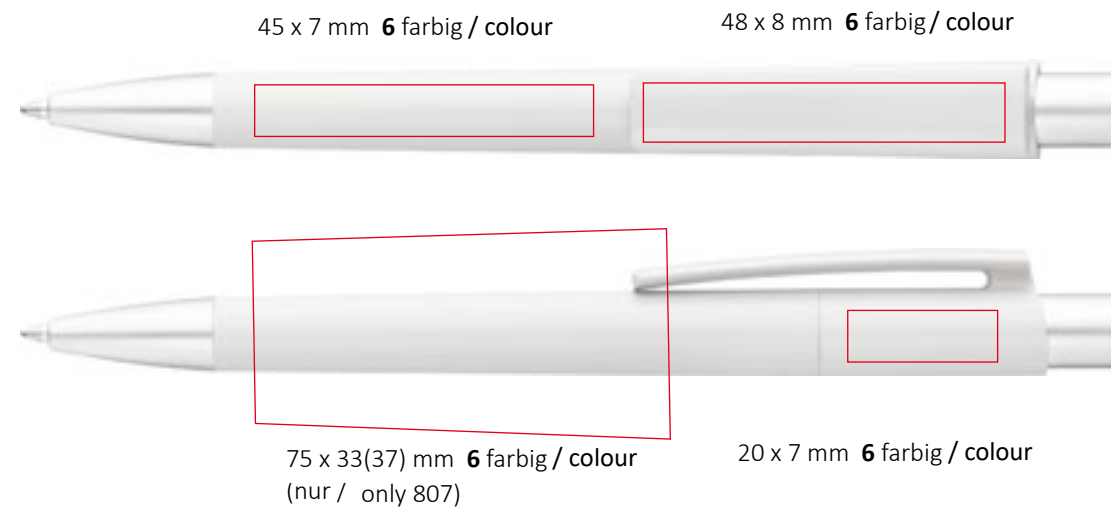
Metallspitze matt 807/808 metal tip matt 807/808
